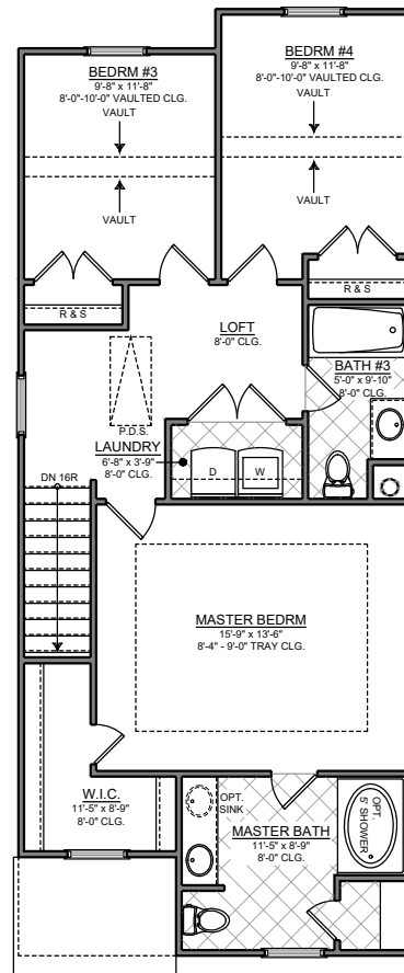
SECOND FLOOR PLAN SCALE: N.T.S
