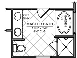
DELUXE MASTER BATH SCALE: N.T.S
