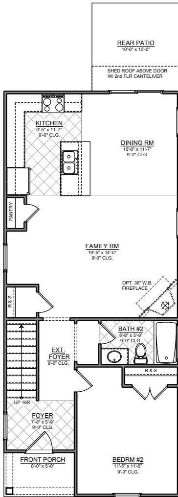
FIRST FLOOR PLAN SCALE: N.T.S
