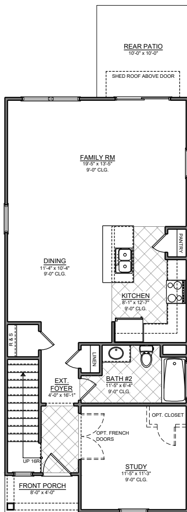
FIRST FLOOR PLAN SCALE: N.T.S
