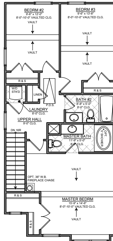
SECOND FLOOR PLAN SCALE: N.T.S
