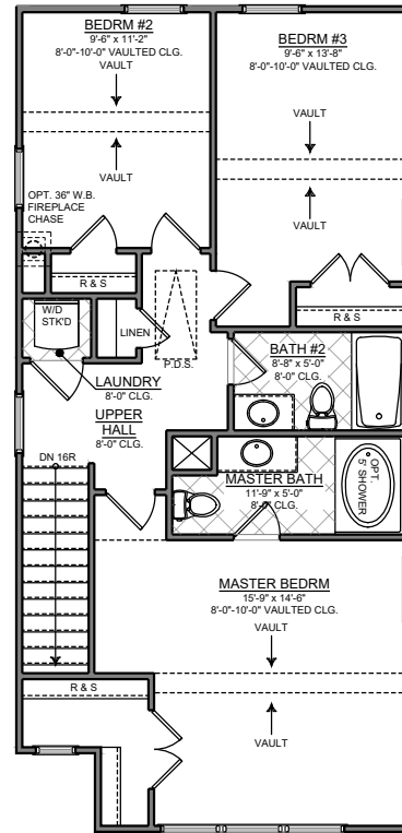
SECOND FLOOR PLAN SCALE: N.T.S
